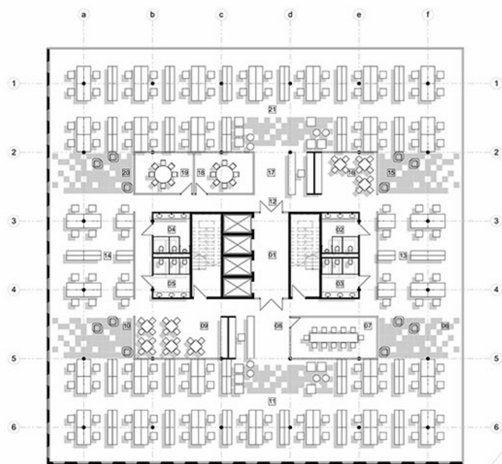
tipinio aukšto planas (I etapas) M 1:250
