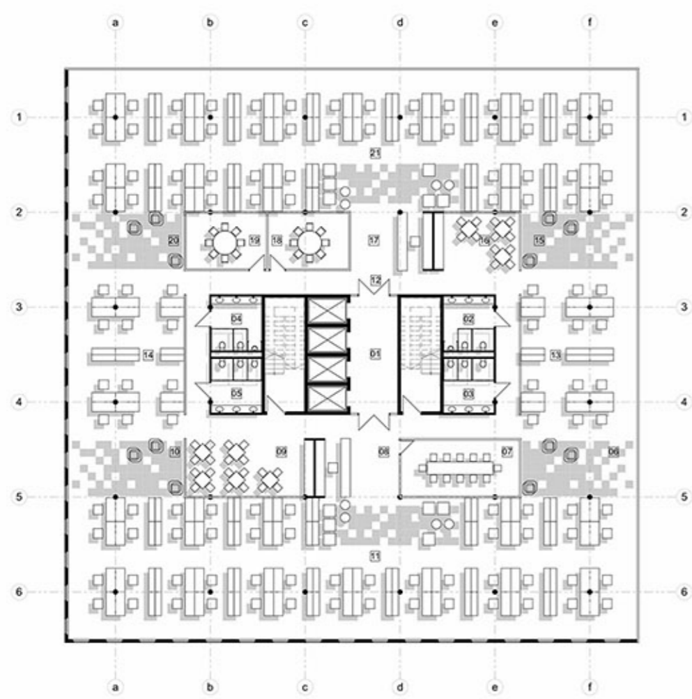
tipinio aukšto planas (II-III etapai) M 1:250
