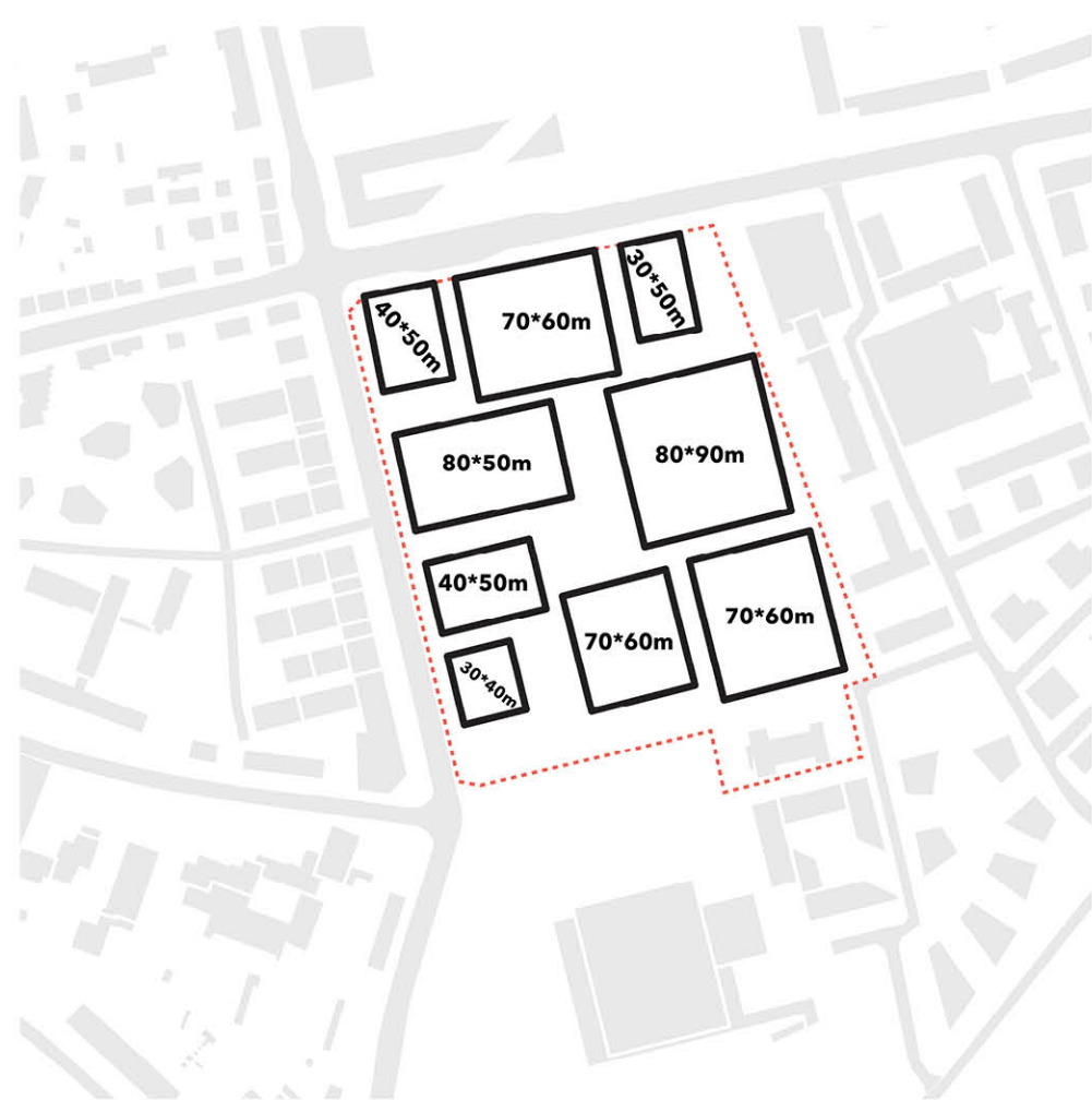
Įvairių dydžių miesto blokai
