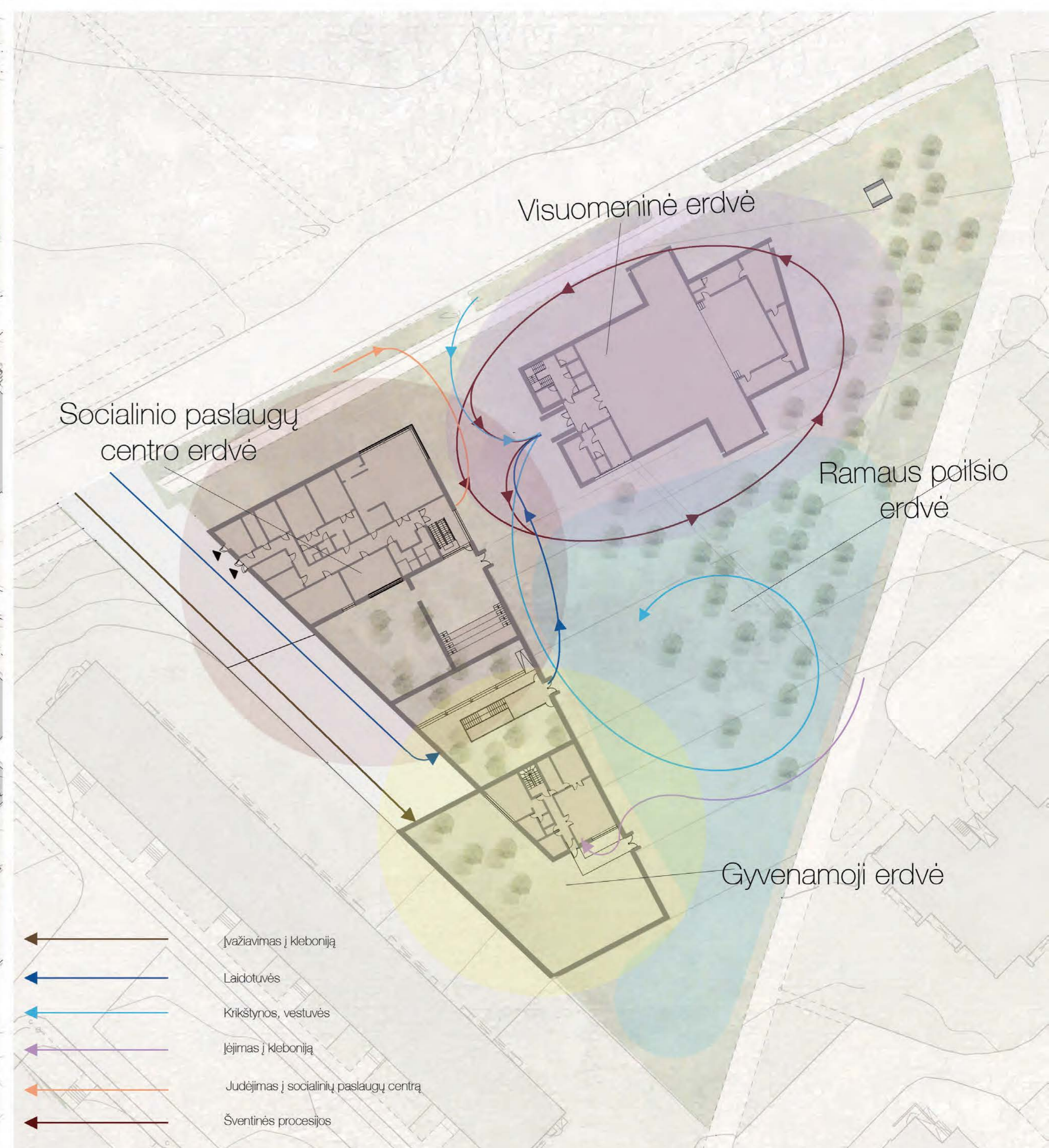
BAŽNYČIOS IR KITŲ PASTATŲ FUNKCINIŲ SRAUTŲ SCHEMA M 1:500
