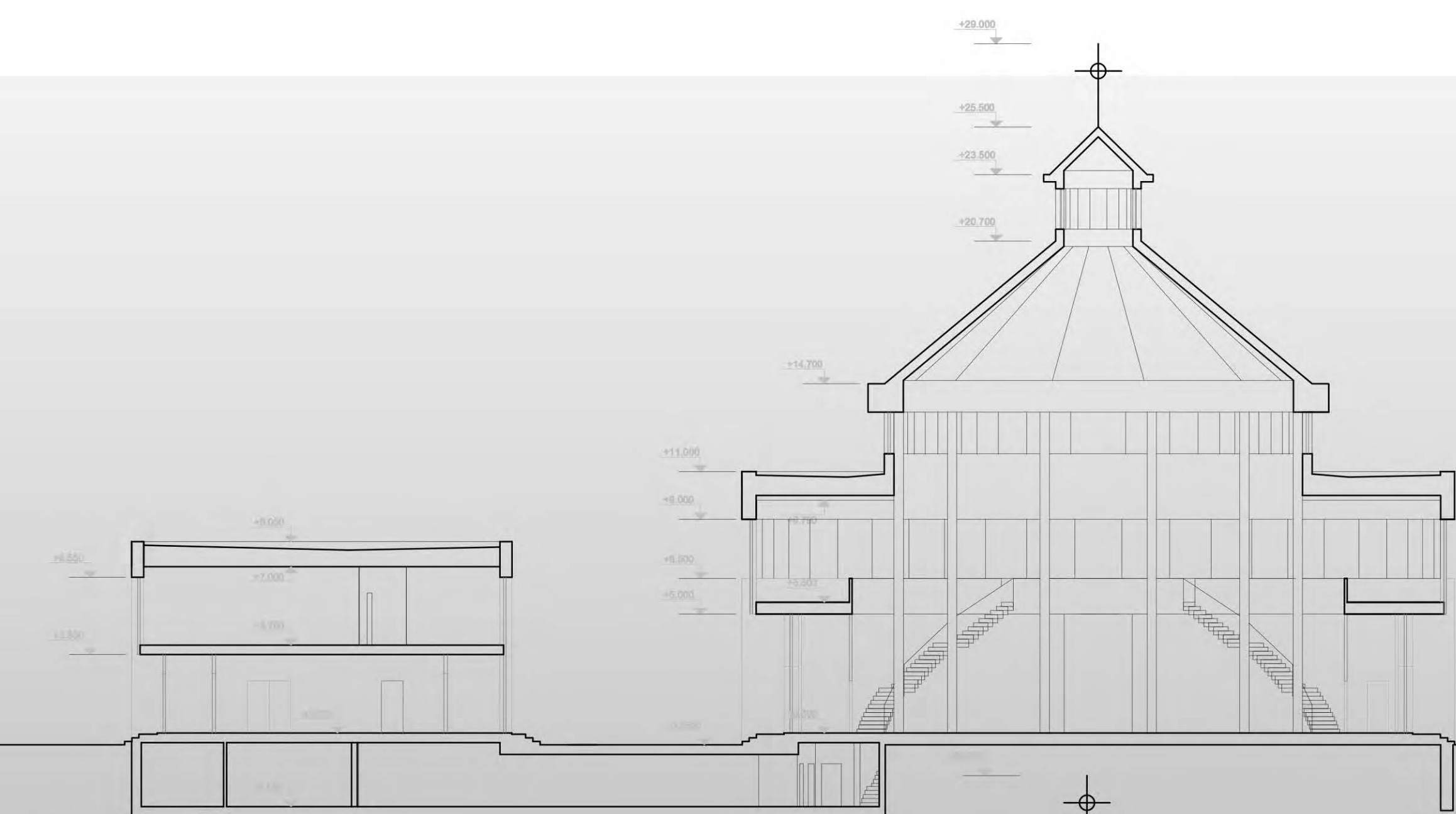
PJŪVIS A-A M1:200
