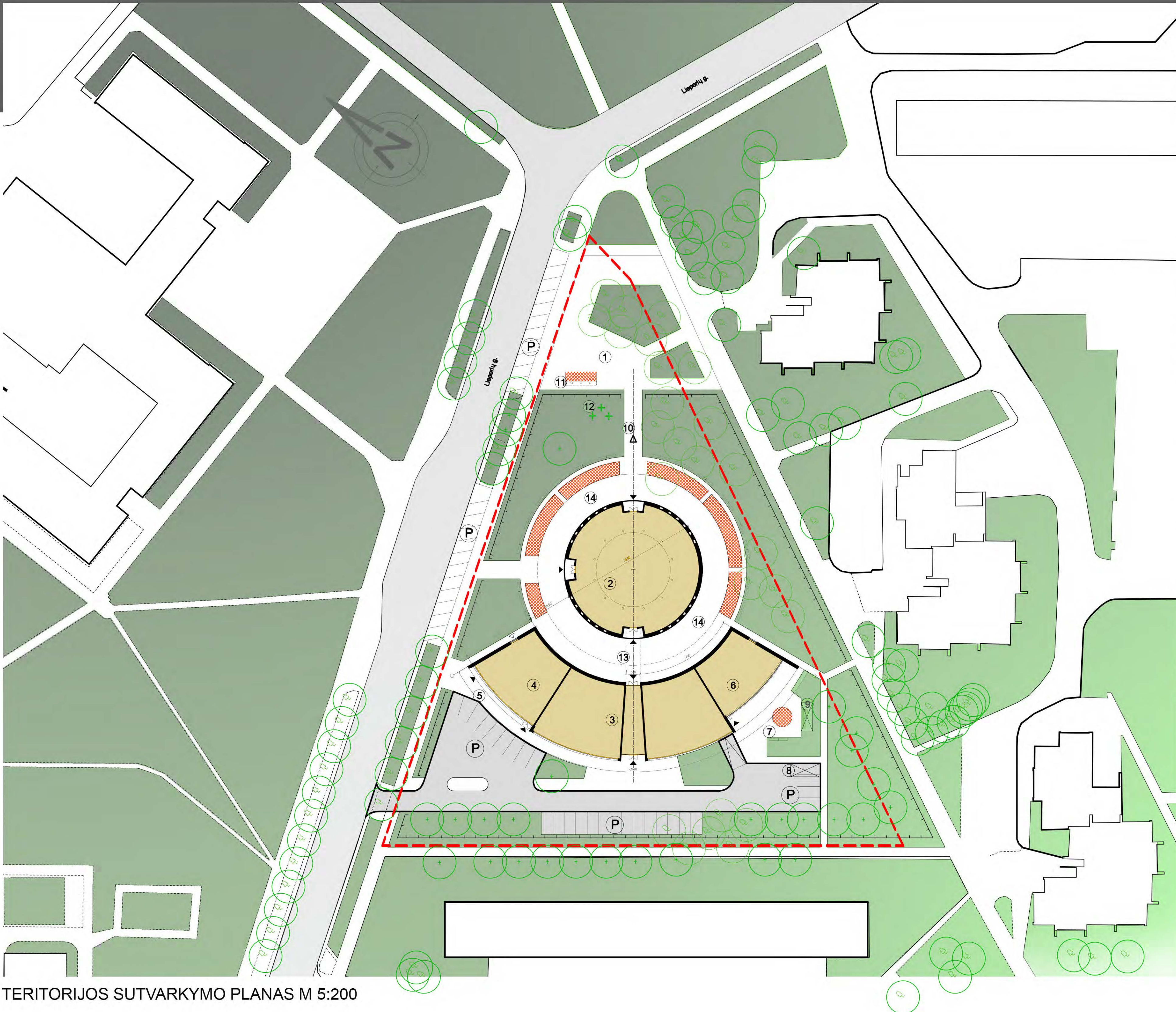
TERITORIJOS SUTVARKYMO PLANAS M 1:500
