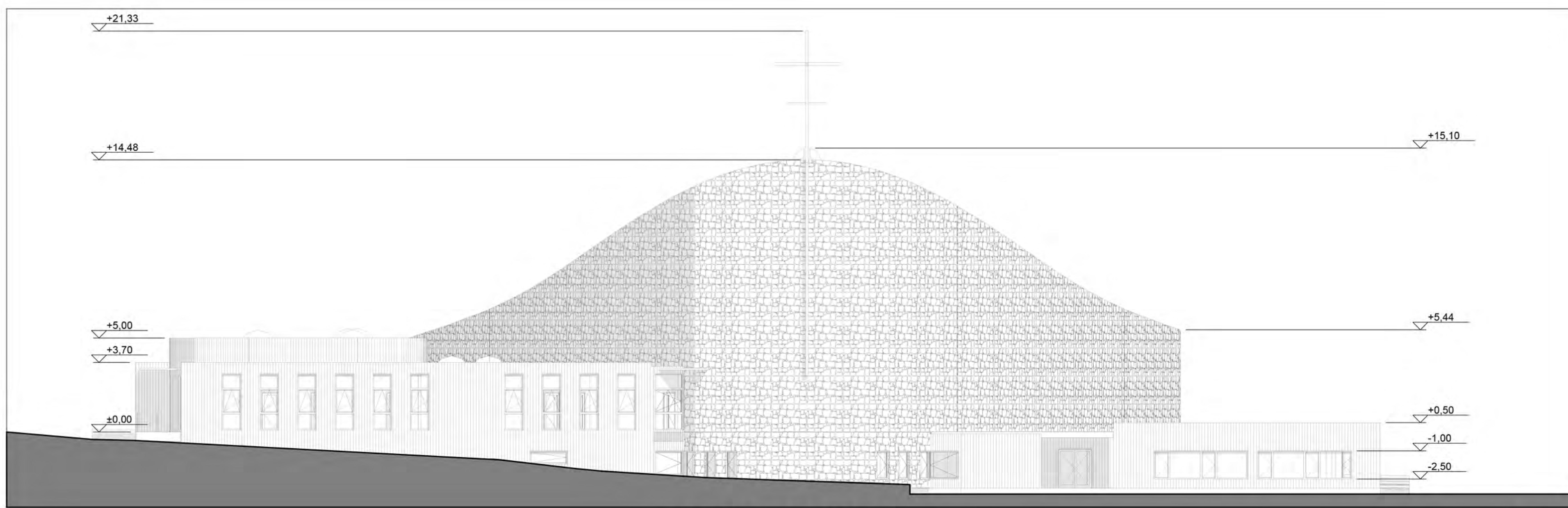
RYTINIS FASADAS
