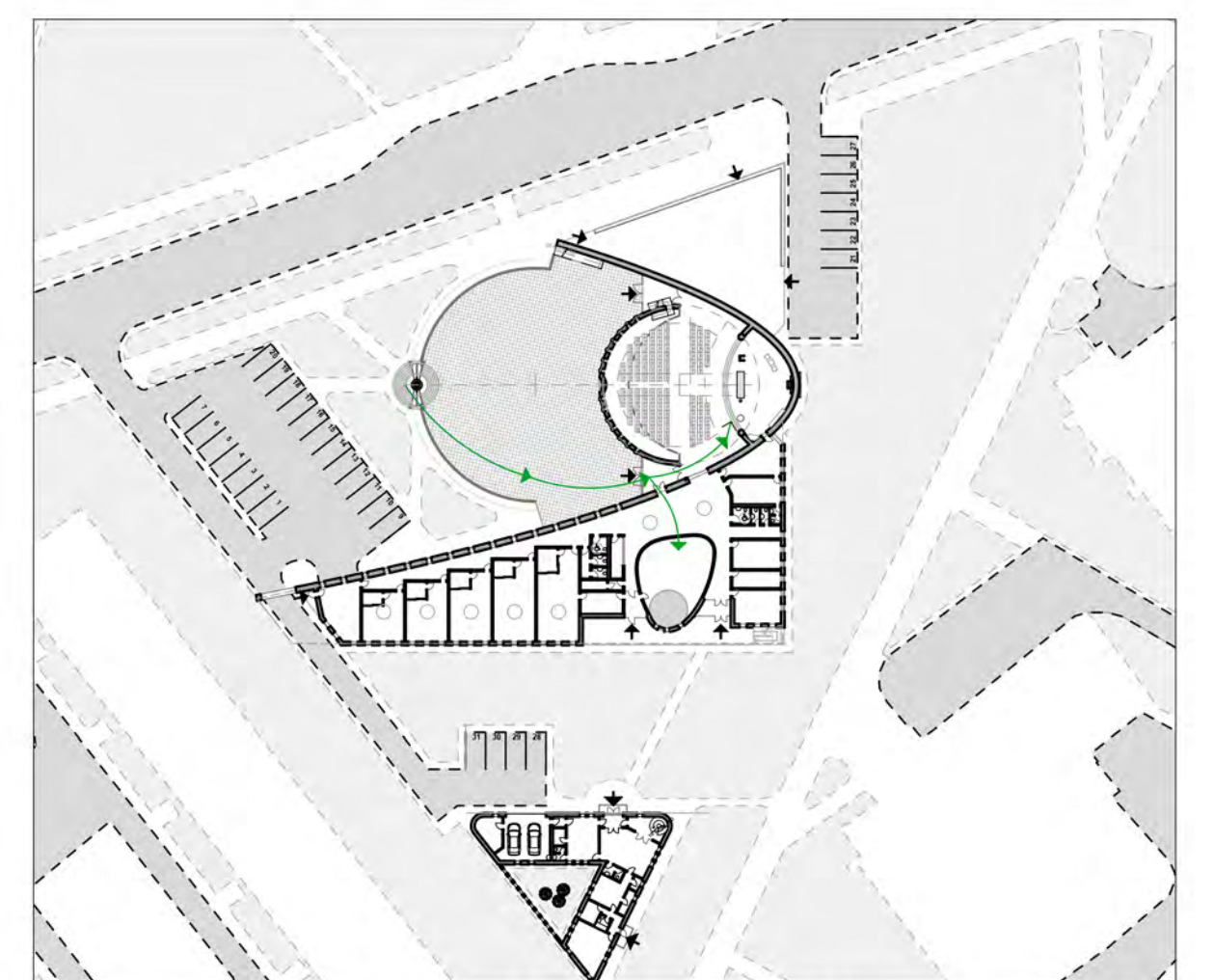
1. KRIKŠTYNŲ SCHEMA 1:1000
