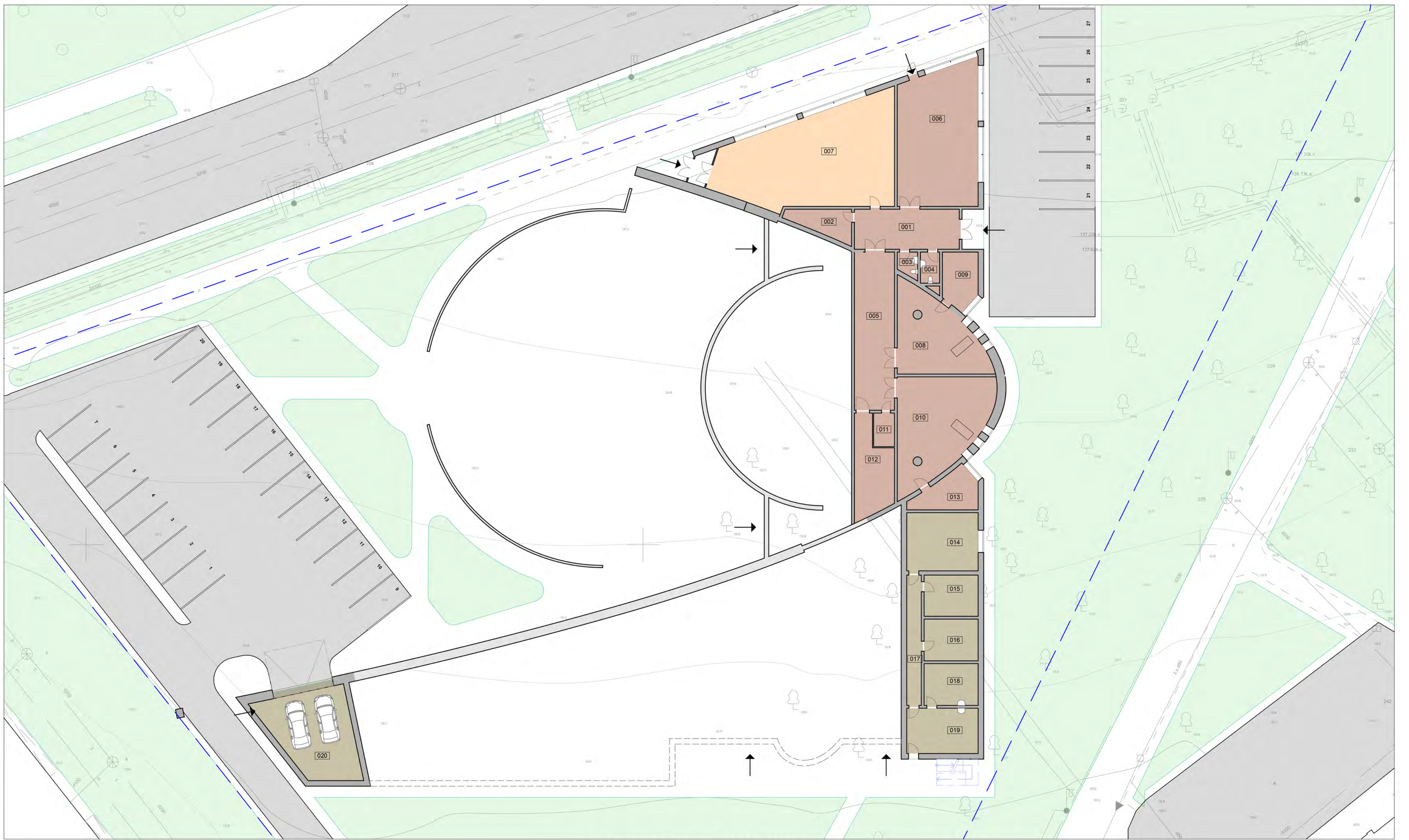
0. COKOLINIO AUKŠTO PLANAS
