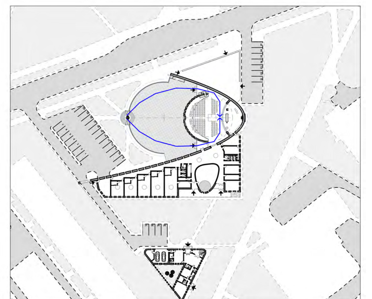
1. VESTUVIŲ SCHEMA 1:1000
