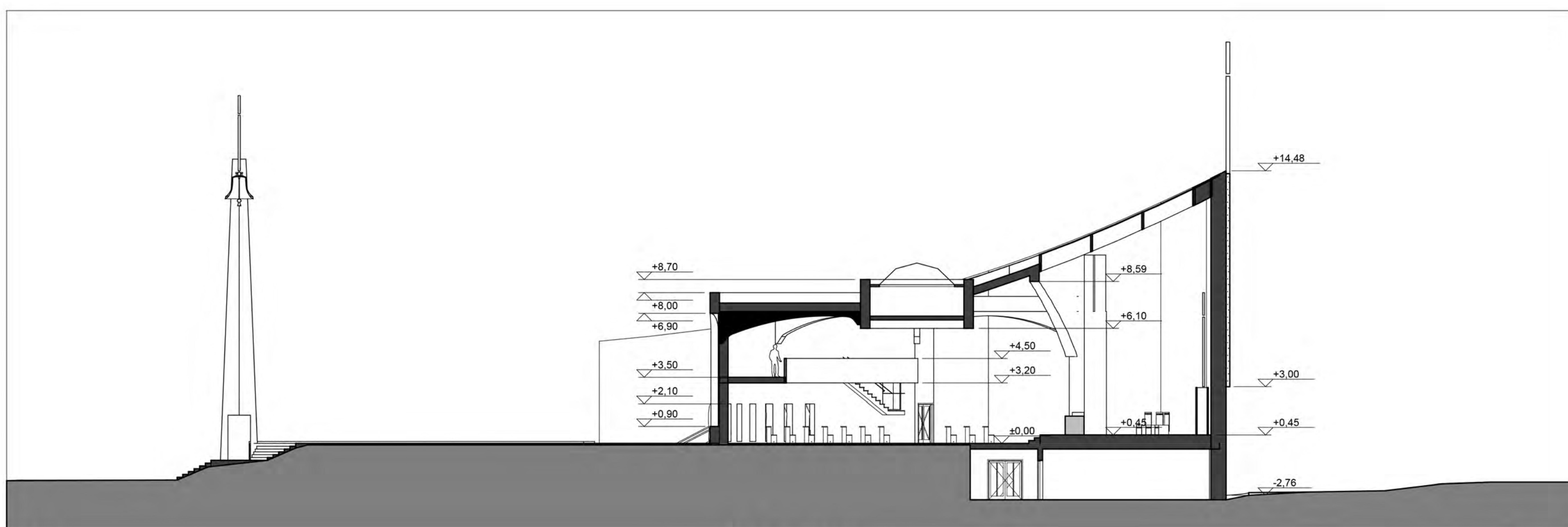
PJŪVIS 2-2
