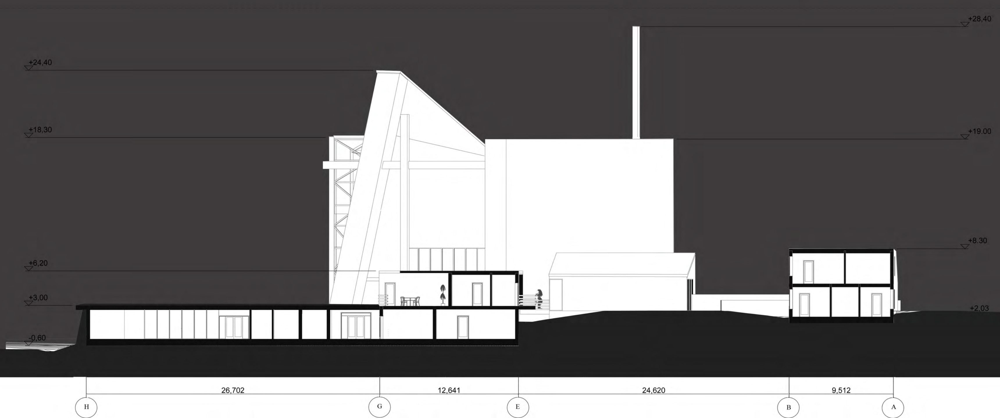
Pjūvis tarp ašiu H-A M1:200
