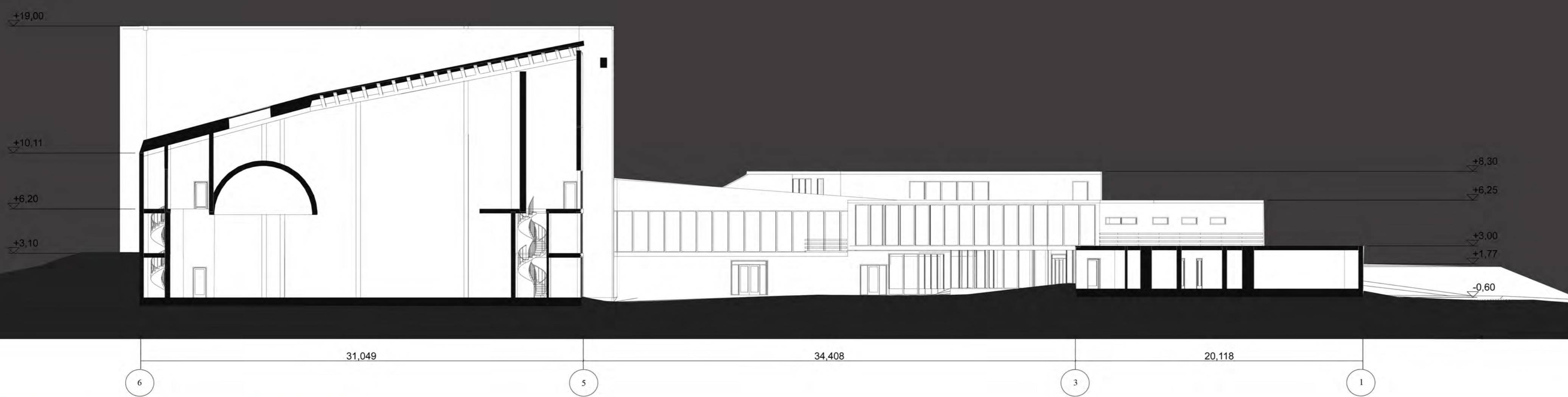
Pjūvis tarp ašių 6-1 M1:200
