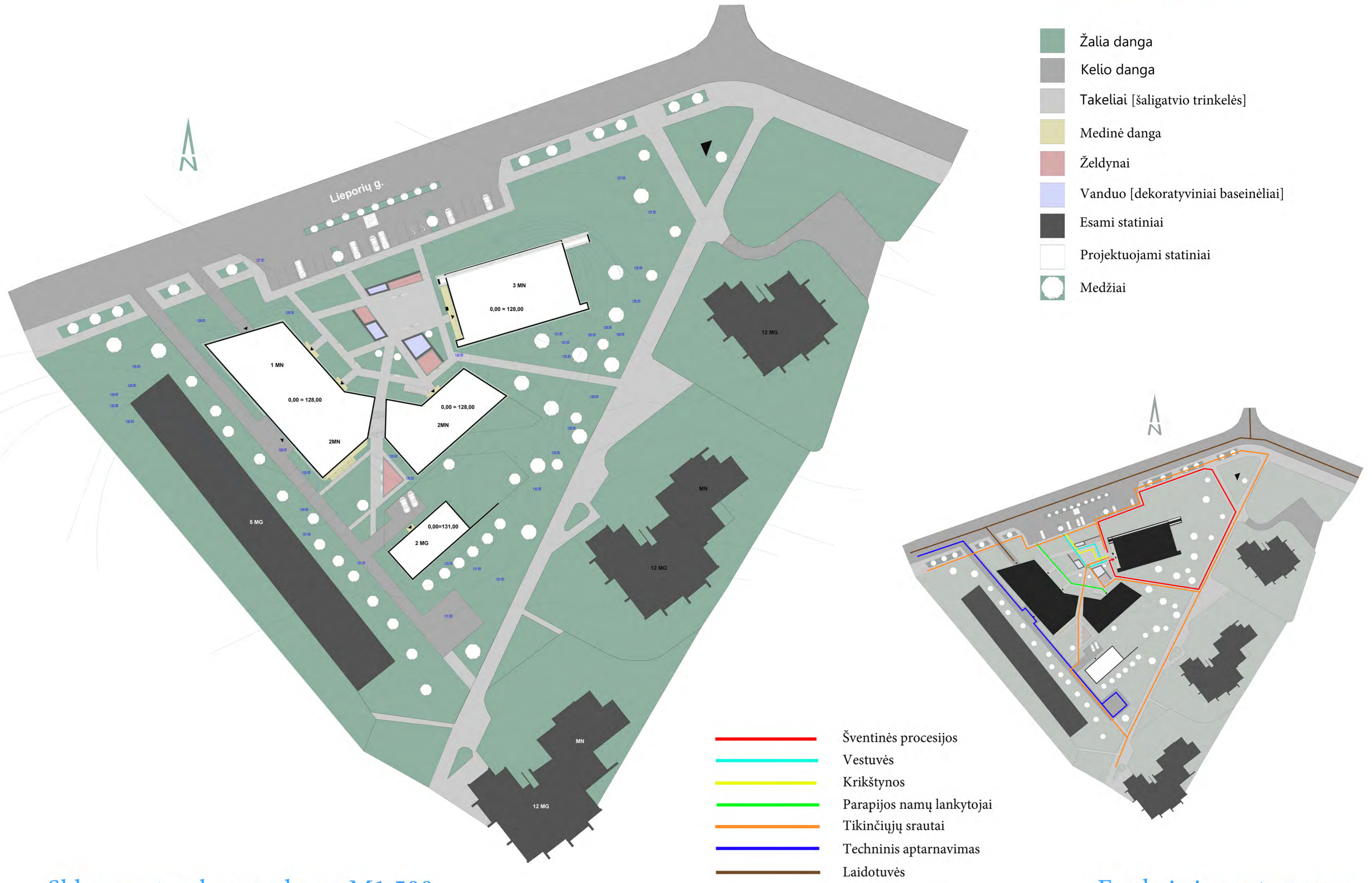
Sklypo sutvarkymo planas M1:500
