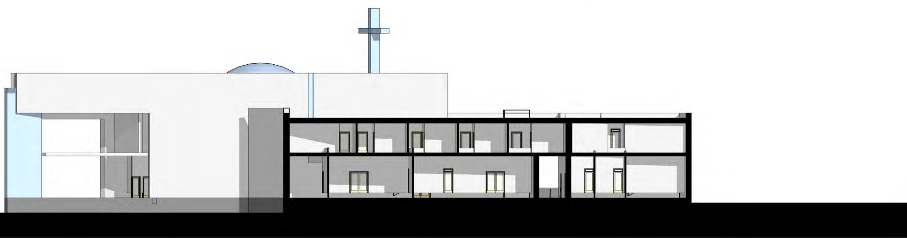
Pietinis fasadas (pjūvis per socialinių paslaugų centrą) m 1:200
