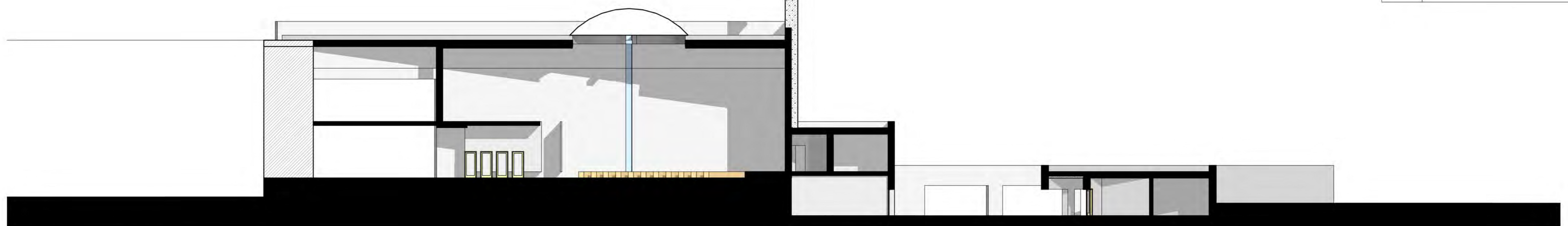
Išilginis pjūvis m 1:200
