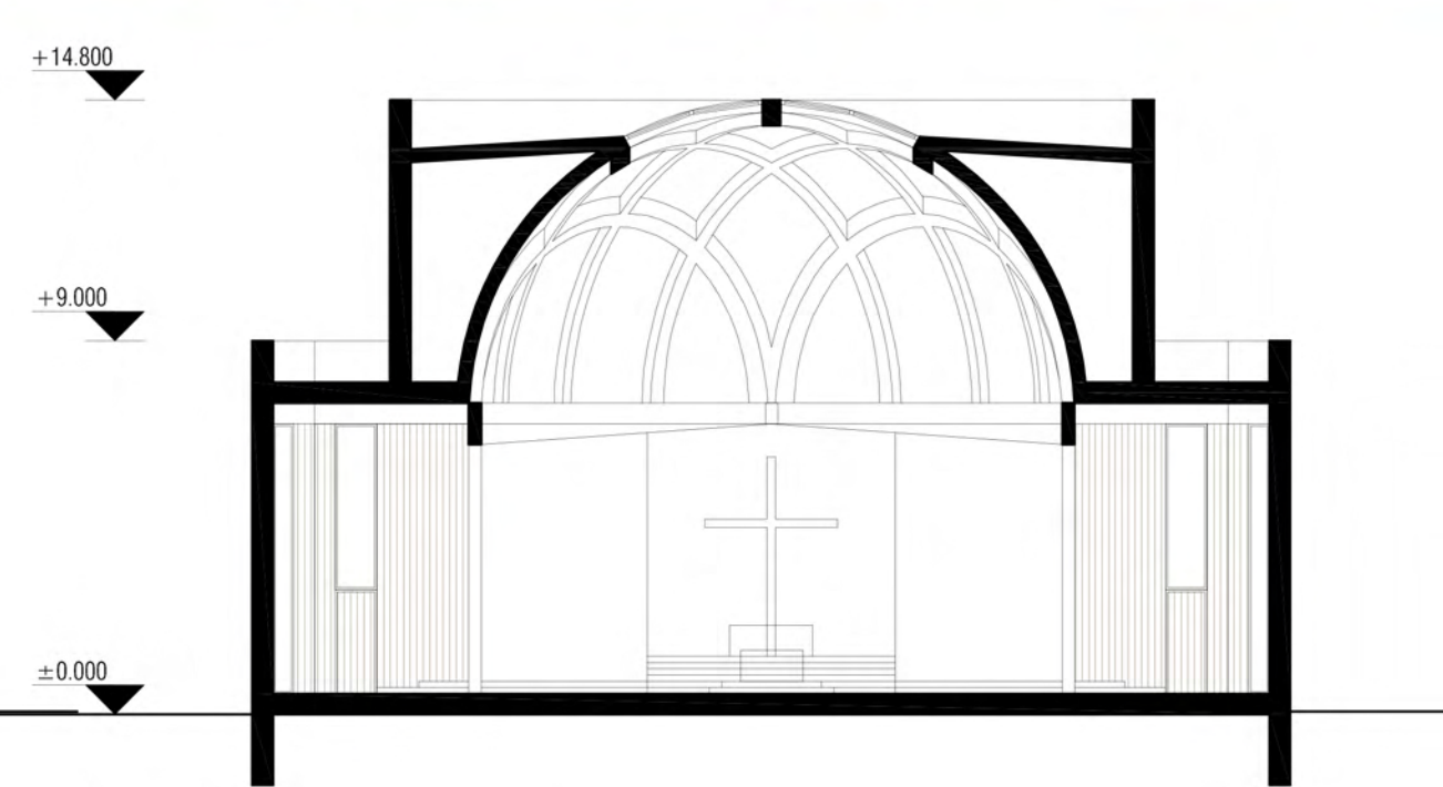
PJŪVIS D-D M 1:200
