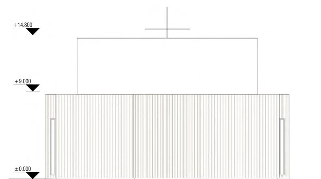
RYTINIS FASADAS D-D M 1:200
