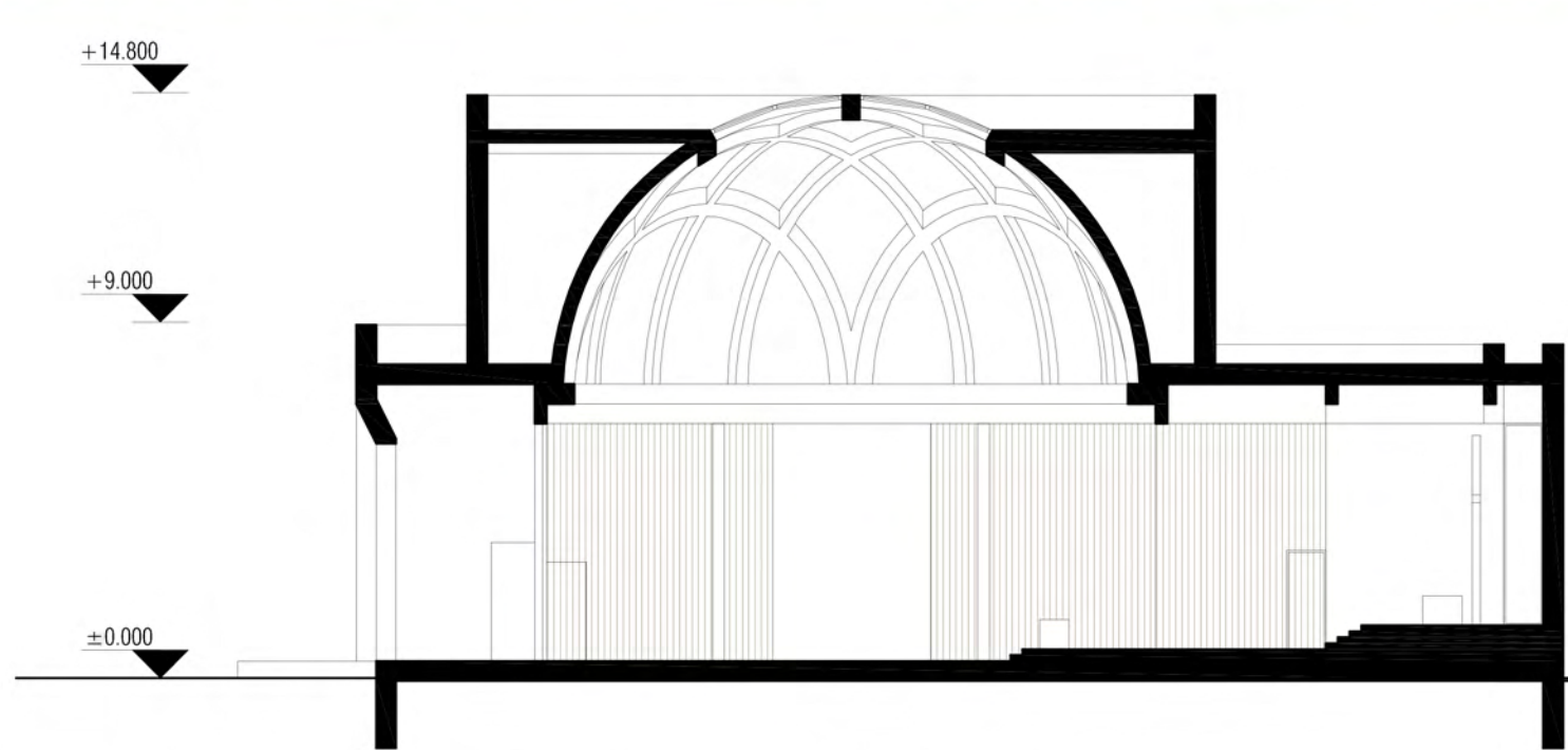
PJŪVIS C-C M 1:200
