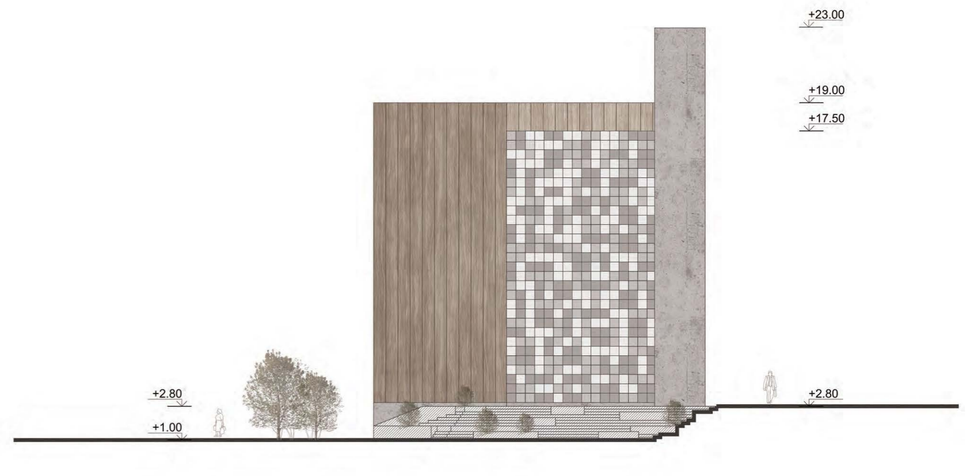
Pietryčių fasadas M 1:200
