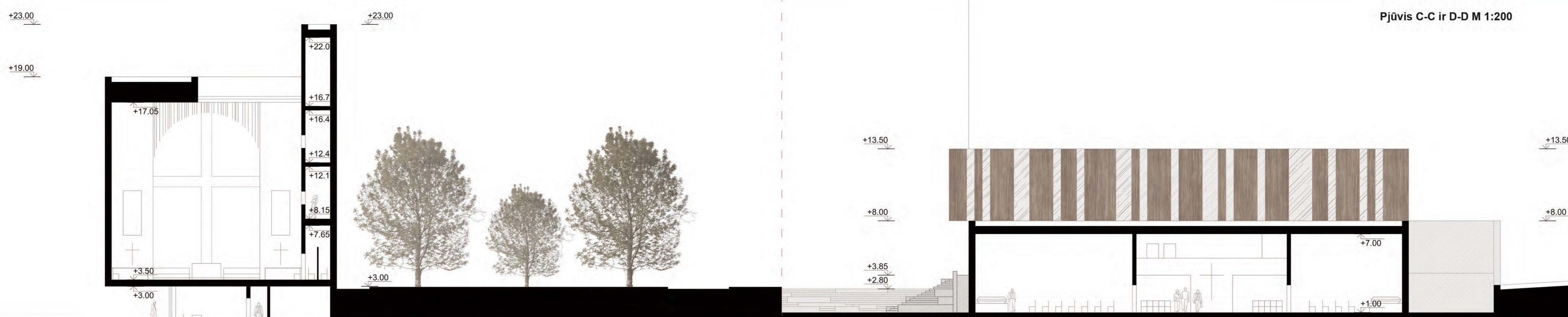
Pjūvis C-C ir D-D M 1:200
