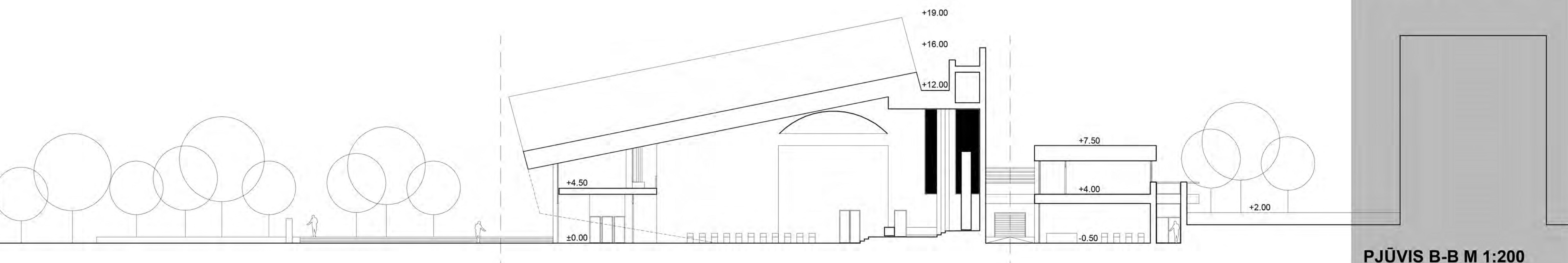
PJŪVIS B-B M 1:200
